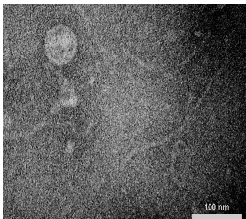
تصویر شماره ۱: تصویر میکروسکوپ الکترونی از فاز پودوویریده با رنگ آمیزی منفی، ۲ درصد اورانیل استات (pH 4-4.5)، ولتاژ 150Kv، با مقیاس 100nm
