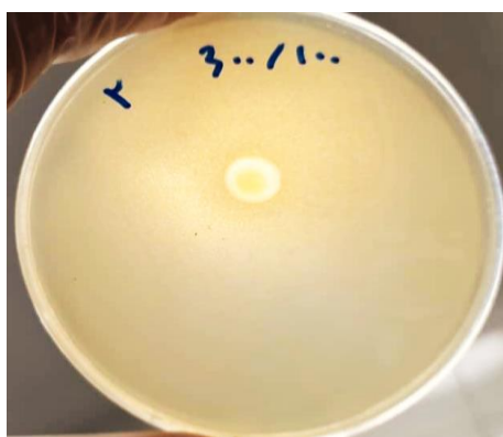
تصویر شماره ۲: روش Spot test، تشکیل هاله عدم رشد و تایید فعالیت لیتیک فاز ایزوله شده علیه هلیکوباکتریپیلوری
