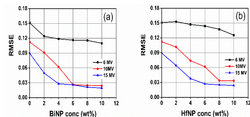
تصویر شماره ۴: مقادیر RMSE در غلظت‌های مختلف از نانوذرات، بیسموت و h: هافنیوم
