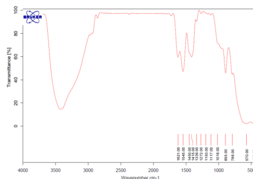
تصویر شماره ۱: طیف FTIR کامپوزیت نانو ذرات مغناطیسی آهن-زیر کونیم/کیتوسان
