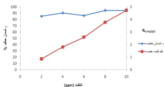
تصویر شماره ۷: مقایسه تغییرات غلظت بر راندمان حذف کروم با استفاده از نانو ذرات مغناطیسی آهن- زیرکونیوم / کیتوسان دمای 25°C، دوز جاذب 2gr/l، سرعت 300 rpm، زمان 60 دقیقه و pH=4
