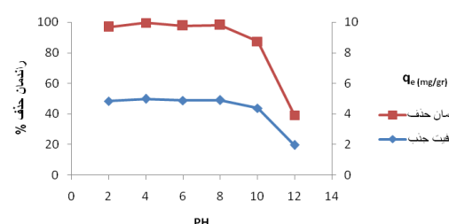
تصویر شماره ۶: مقایسه اثر تغییرات pH بر راندمان حذف کروم با استفاده از نانو ذرات مغناطیسی آهن- زیرکونیوم / کیتوسان غلظت 5ppm Cr^{6+} ، سرعت 300 rpm، زمان 30 دقیقه، دمای 25°C و دوز جاذب 1 g/l
