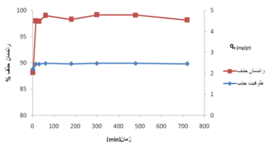
تصویر شماره ۵: مقایسه تغییرات زمان تماس بر راندمان حذف کروم با استفاده از نانو ذرات کیتوزان- زیرکونیوم- آهن غلظت 5ppm Cr^{6+} ، دوز جاذب 2g/l، سرعت 200rpm، دمای 25°C و pH=4
