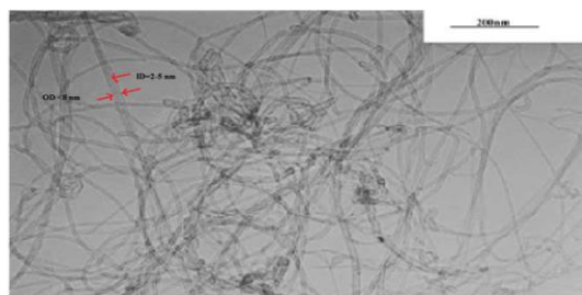
تصویر شماره ۳: تصویر TEM نانولوله های کربنی اصلاح نشده
