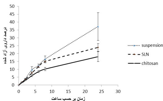
نمودار شماره ۷: مقایسه آزاد سازی داروی اسپرونولاکتون از سه فرم نانوسپانسیون، نانوذرات لیپیدی جامد و نانوذرات روکش شده با کیتوسان در محیط انحلال در زمان‌های مختلف
