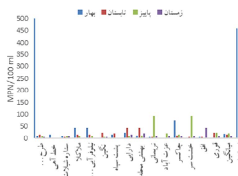
نمودار شماره 2: مقایسه آلودگی کلیفرم‌های مدفوعی در 15 ایستگاه نمونه برداری شهرستان محمودآباد در 4 فصل مختلف با استاندارد
