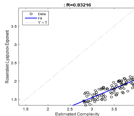
نمودار شماره 4: نمودار رگرسیون بین سری زمانی نمای لیپانف با روش Rosenstein و پیچیدگی تخمین زده شده
