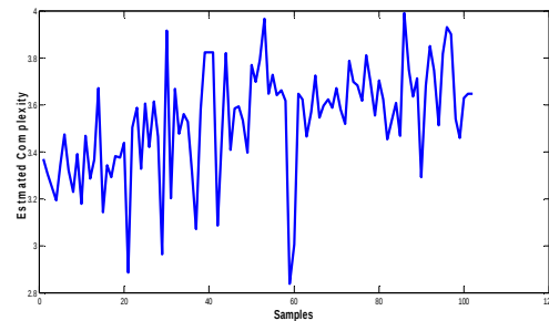
نمودار شماره 2: سری زمانی پیچیدگی تخمین زده شده
