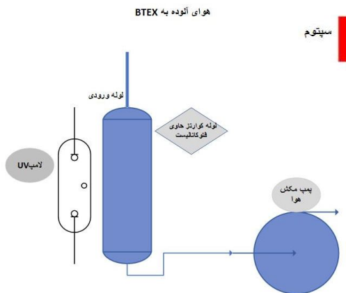
تصویر شماره 1: تصویر و شماتیک پایلوت آزمایشگاهی ساخته شده سیستم مورد آزمایش
