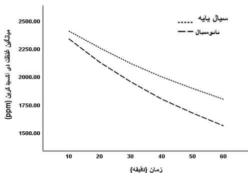
تصویر شماره 5: ارتباط بین سیال پایه و نانوسیال با میزان جذب دی اکسید کربن
