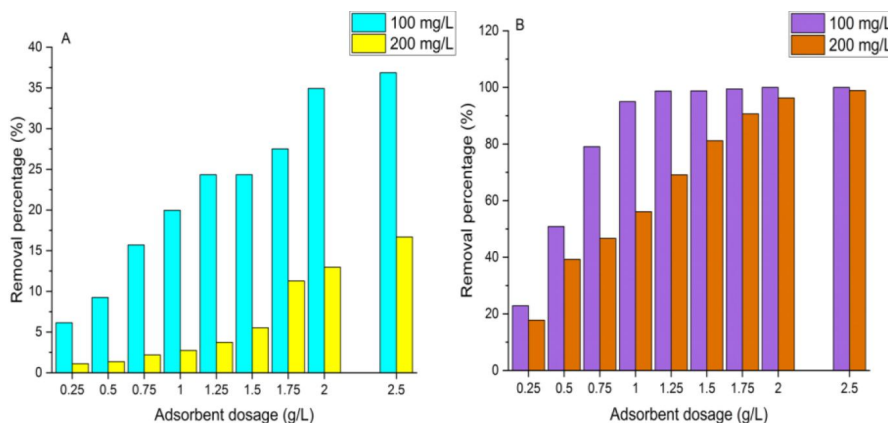
تصویر شماره 4: بررسی اثر دوز جاذب بر روی کارایی جذب AR-18 (A)؛ نانو ذرات MgO و PAC؛ شرایط آزمایش: زمان تماس دو ساعت، دمای 20 درجه سلسیوس و pH طبیعی محلول)
