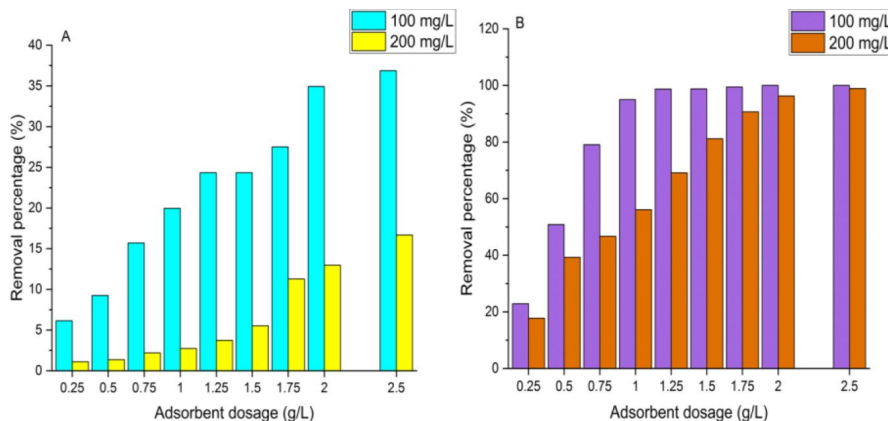
تصویر شماره 4: بررسی اثر دوز جذب بر روی کارایی جذب AR-18 (A) نانو ذرات MgO و PAC؛ شرایط آزمایش: زمان تماس دو ساعت، دمای 20 درجه سلسیوس و pH طبیعی محلول)
