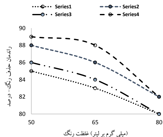
نمودار شماره ۱: اثر غلظت اولیه رنگ و مقدار لجن بر راندمان حذف رنگ در دو حالت هوازی و بی‌هوازی در زمان ۸ روز
