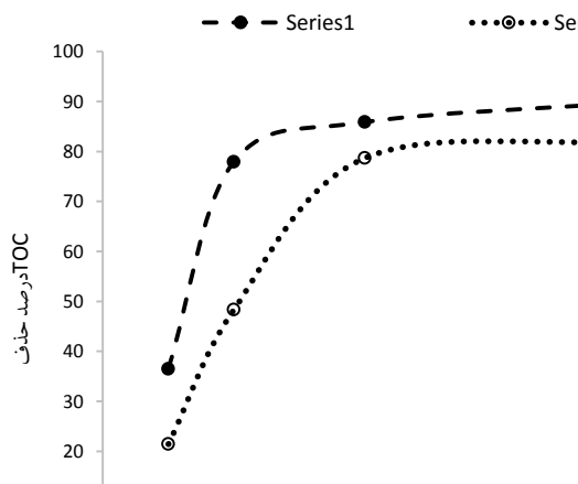
نمودار شماره ۴: تاثیر زمان تماس بر حذف TOC در دو حالت هوازی و بی هوازی
