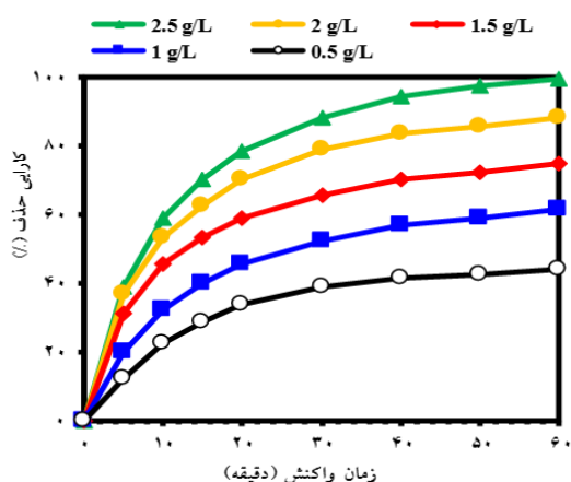
نمودار شماره ۵: تأثیر مقدار اولیه نانو کامپوزیت بر کارایی حذف سونو کاتالیستی دیازینون (غلظت اولیه دیازینون برابر با ۲۰ mg/L، pH اولیه برابر با ۵)
