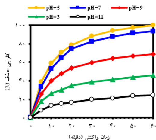
نمودار شماره ۴: تأثیر pH اولیه بر کارایی حذف سونو کاتالیستی دیازینون (غلظت اولیه دیازینون برابر با ۲۰ mg/L، مقدار اولیه نانو کامپوزیت برابر با ۲/۵ g/L)
