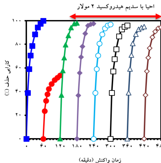
نمودار شماره ۱۳: کارایی نانو کامپوزیت بازیافت شده بر حذف سونو کاتالستی دیازینون (غلظت اولیه‌ی دیازینون برابر با ۲۰ mg/L، مقدار اولیه‌ی نانو کامپوزیت برابر با ۲/۵ g/L، pH اولیه برابر با ۵)
