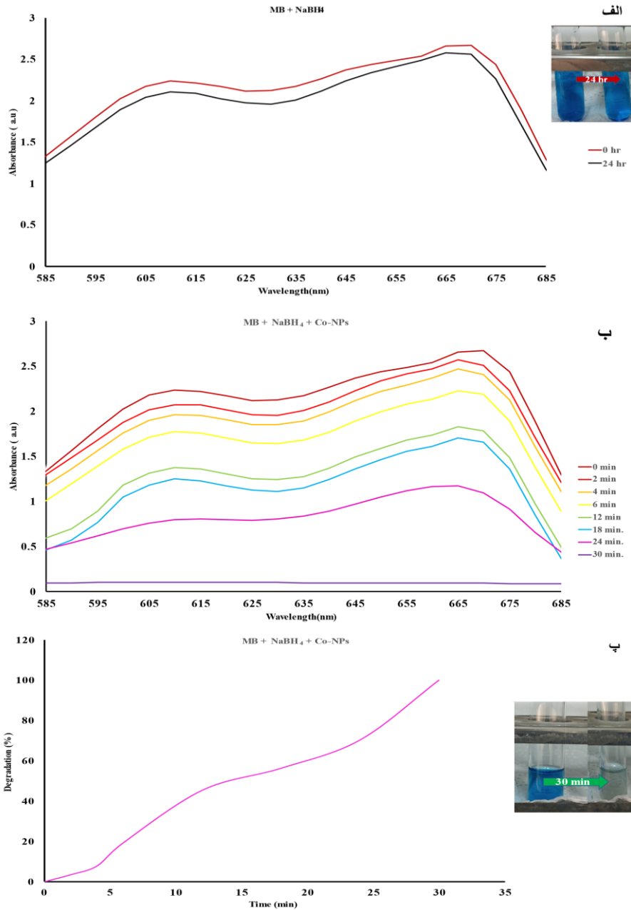
نمودار شماره ۵: الف) میزان رنگبری متیلن بلو در حضور NaBH 4 بدون نانوذرات، ب) فعالیت فتوکاتالیستی نانوذرات کبالت در جهت تخریب MB در حضور NaBH 4 ، پ) درصد تخریب رنگ MB در گذر زمان در حضور نانوذرات کبالت
