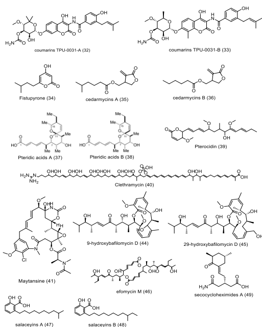
تصویر شماره ۲: ساختار شیمیایی پلی کتیدها
