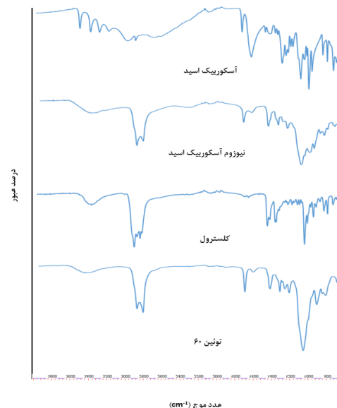
تصویر شماره ۳: طیف های ATR-FTIR آسکوربیک اسید، نیوزوم آسکوربیک اسید (F10)، کستروال و توتین ۶۰
