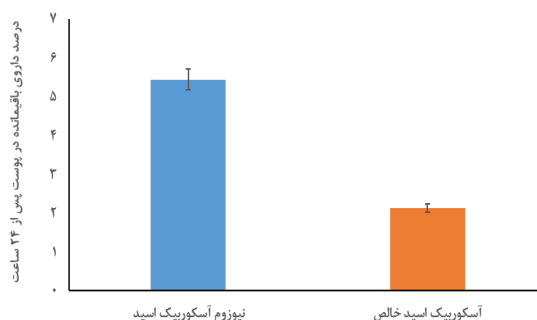
تصویر شماره ۷: میزان آسکوربیک اسید باقیمانده در پوست از نیوزوم (F10) در مقایسه با محلول دارو پس از پایان آزمون جذب پستی
