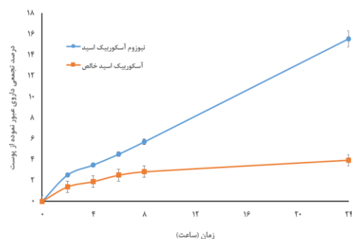
تصویر شماره ۶: روند جذب پستی آسکوربیک اسید از نیوزوم (F10) در مقایسه با محلول دارو از خلال پوست ناحیه شکمی رت با استفاده از سلول فرانز
