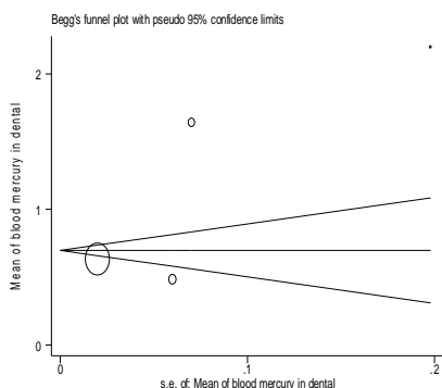
نمودار شماره B.6. سوگرایی انتشار برای مطالعات مرتبط با میانگین غلظت جیوه در نمونه خون (P=0/304).
