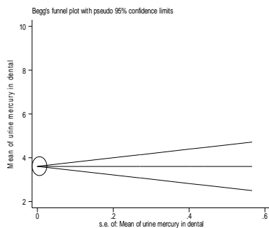
نمودار شماره A.6. سوگرایی انتشار برای مطالعات مرتبط با میانگین غلظت جیوه در نمونه ادرار (P=0/096).
