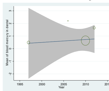
نمودار شماره B.5. متارگرسیون میانگین جیوه در نمونه خون برحسب سال انجام مطالعه. دایره های بزرگ تر، حجم نمونه بزرگتر را نشان می دهند (P=0/581).
