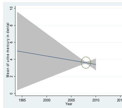
نمودار شماره A.5. متارگرسیون میانگین جیوه در نمونه ادرار برحسب سال انجام مطالعه. دایره های بزرگ تر، حجم نمونه بزرگتر را نشان می دهند (P=0/265).
